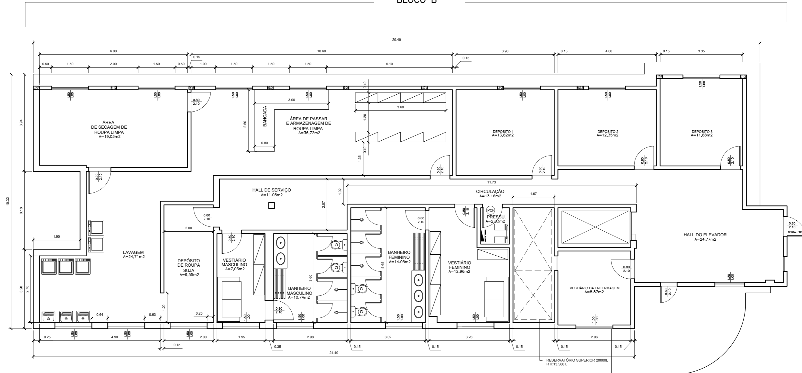
PLANTA BAIXA – 5º PAVIMENTO – BLOCO B – PROPOSTO
